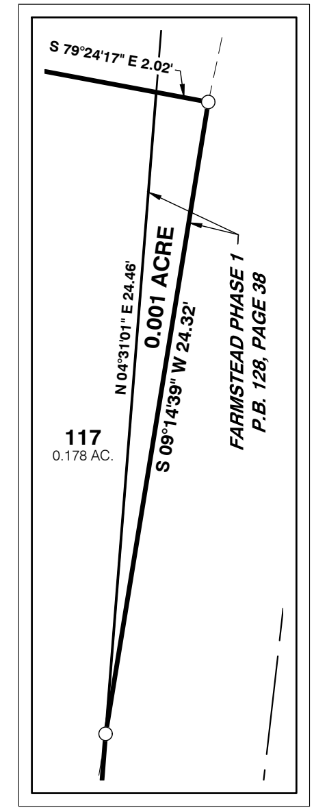
DETAIL "B" SCALE: 1" = 5'
